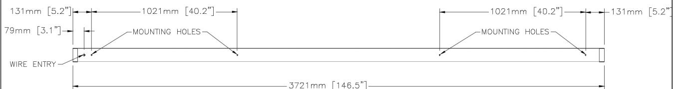
12FT LUMINAIRE
