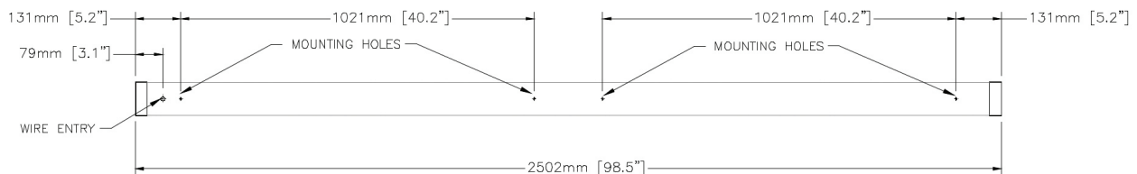
8FT LUMINAIRE
