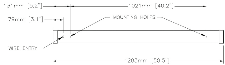
4FT LUMINAIRE
