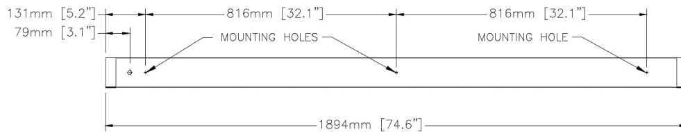
6FT LUMINAIRE
